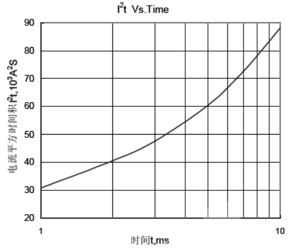
特性曲线
