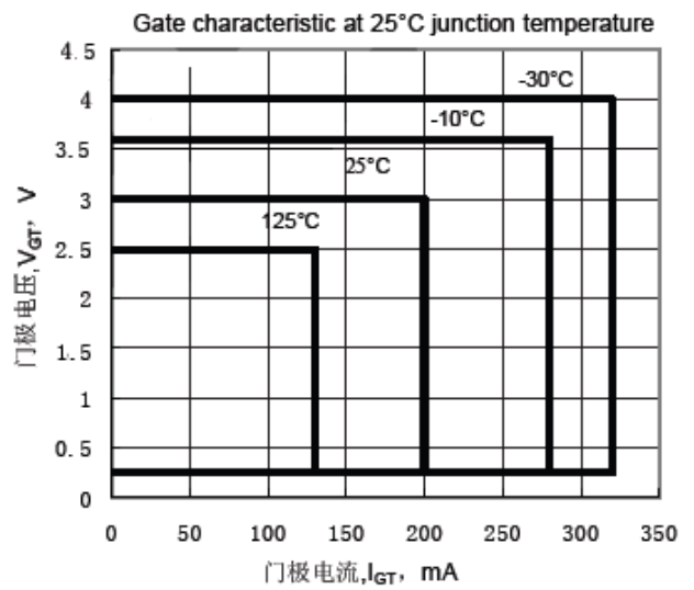
Fig.10 门极触发
