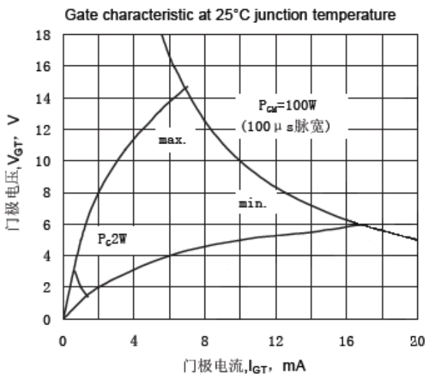
Fig.9 门极功率
