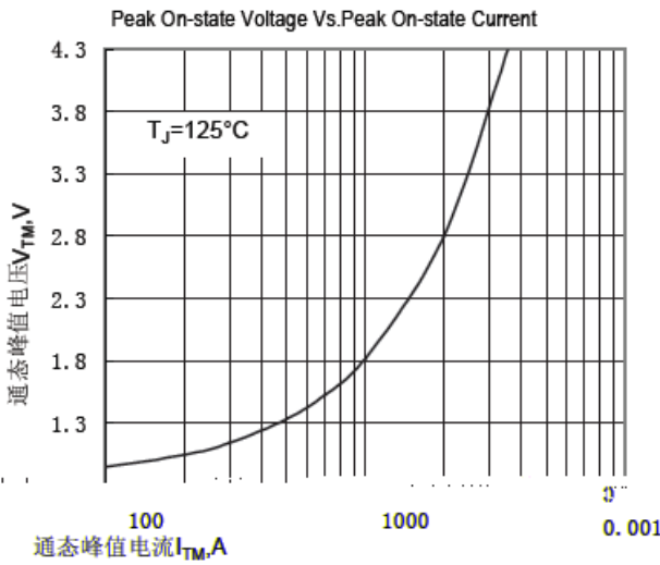
安特性曲线
