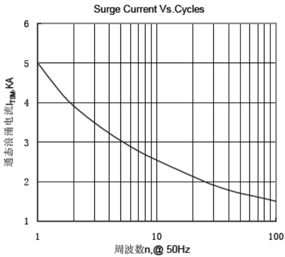
浪涌电流与周波数的关系曲线
